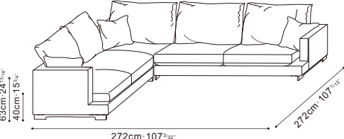
C0150025 + C0150033 + C0150026
